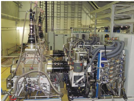
IFMIF RF System, Rokkasho, Japan
