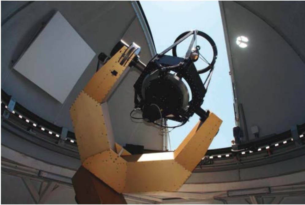
CESAR Project Telescope, ESA-Cebreros
