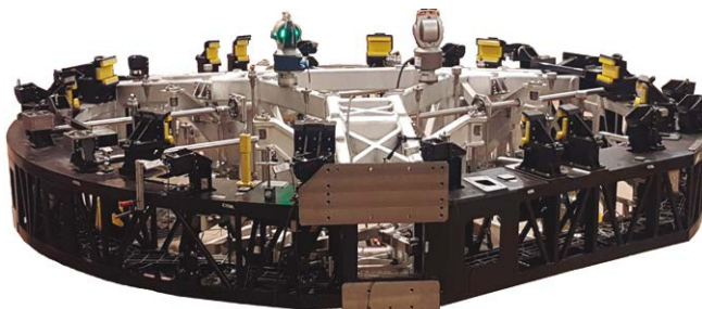
ELT M2 Cell
